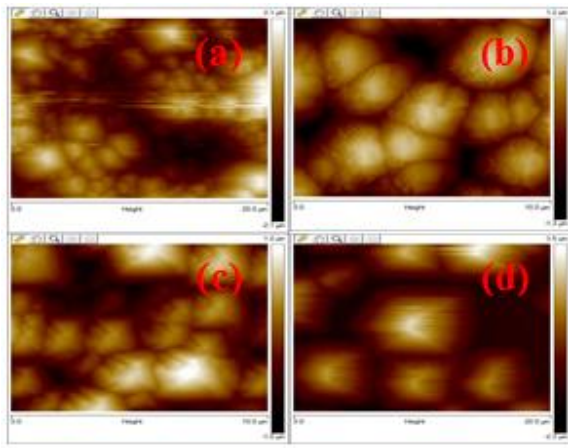
Fig. 3: 2 D Profile AFM Images of KOH Textured Silicon Wafer Samples for (A) 30 Min, (B) 40 Min, (C) 50 Min and (D) 60 Min.
