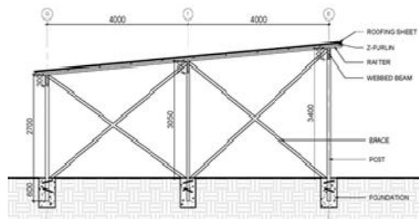
Fig. 4:Longitudinal Section.
