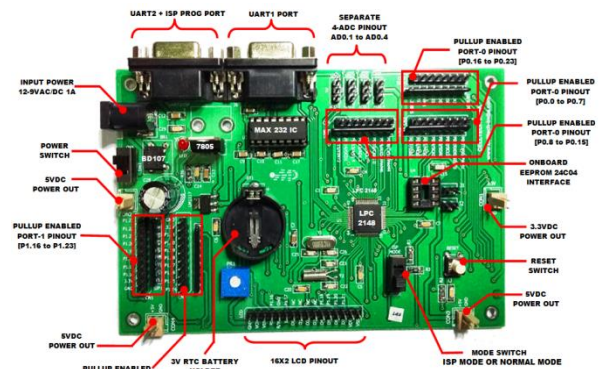
Fig. 2: ARM 7 LPC 2148.
