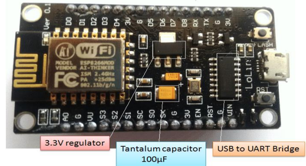
Fig. 2: NodeMCU Microcontroller.
