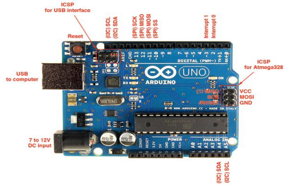
Fig. 3: The Arduino UNO Microcontroller.
