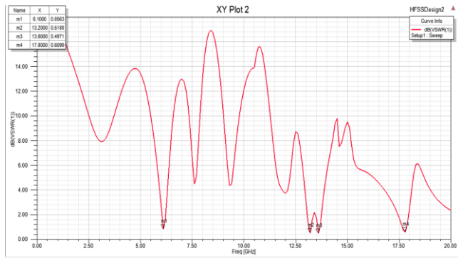
Fig. 4 VSWR Values
