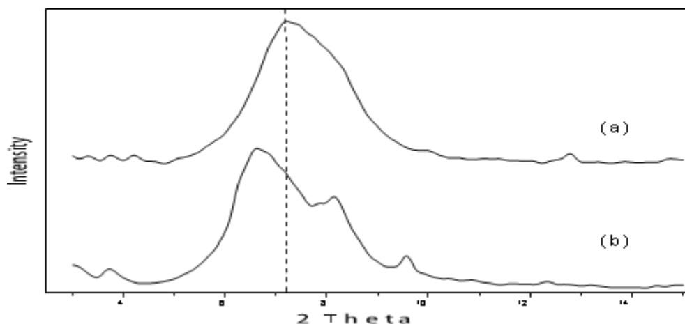
Fig. 1: XRD Patterns of (A) \text{Na}^+ -MMT, (B) Ce (IV) -MMT.
