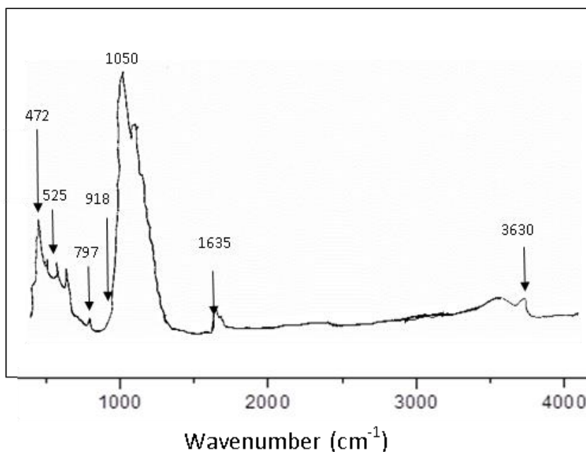
Fig. 3: FT-IR Spectrum for Na + -MMT.
