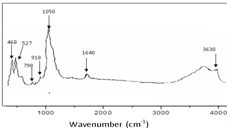
Fig. 3: FT-IR Spectrum for Na + -MMT.
