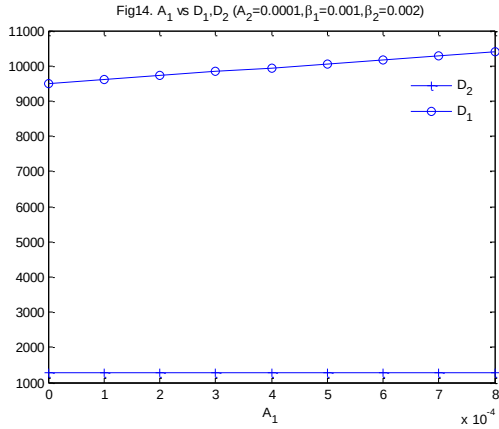
Fig. 14: A1 Vs D1, D2 for A2=0.0001, B1=0.001, B2=0.002
